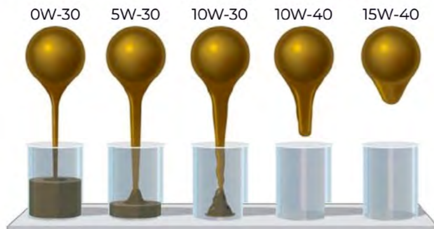
Вязкость различных масел при температуре -20°C
