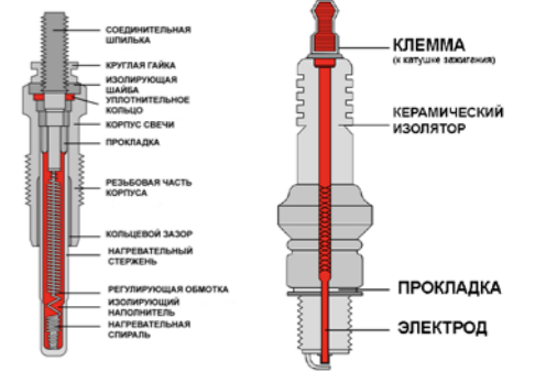
СВЕЧА ЗАЖИГАНИЯ СВЕЧА НАКАЛИВАНИЯ
